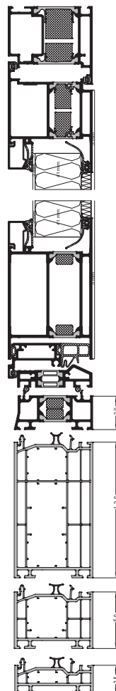
Bodenanschluss- profile
