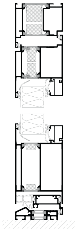
Standardtür mit Einsatzfüllung
